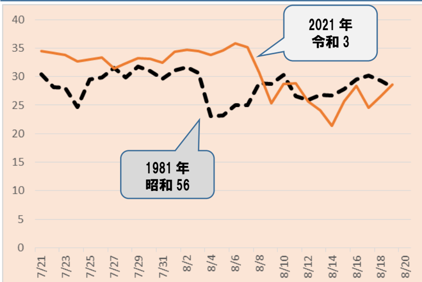
夏の最高気温比較（奥出雲町横田 1981年・2021年 7月21日～8月19日）
